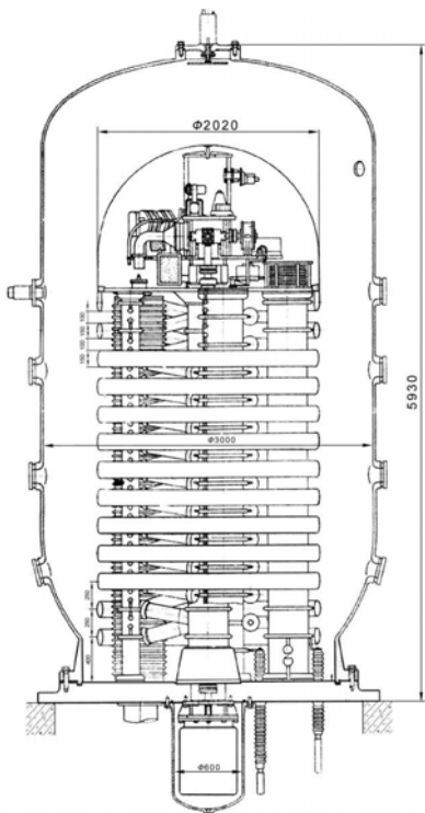
Рис. 5. Высоковольтная структура ускорителя КГ-2,5.
