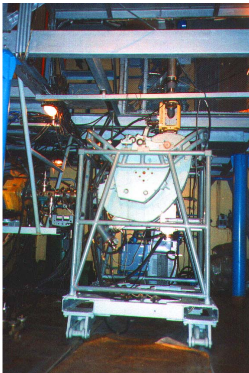
Рис. 6. Электромагнитный масс-анализатор.
