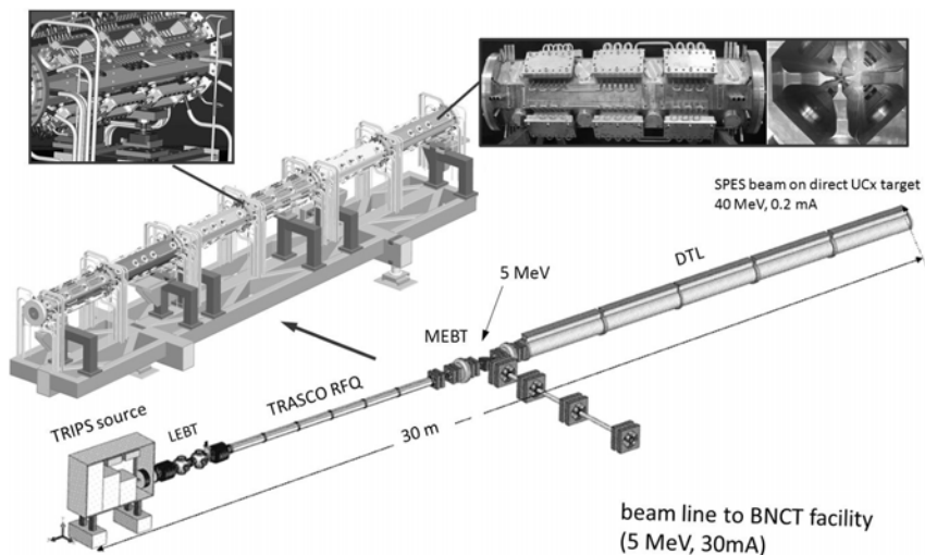
Рис. 4. Схема установки SPES-1.
