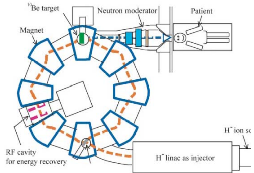
Рис. 9. Схема установки ERIT.
