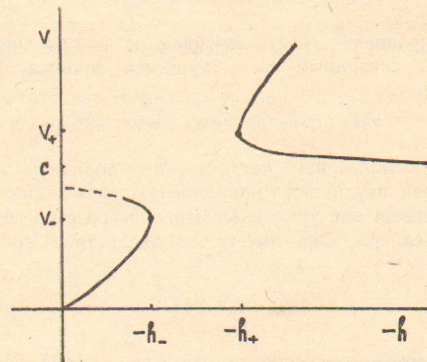
Рис. 1. Зависимость скорости движения фронта фазового перехода от внешнего поля. Штриховой линией отмечена область, в которой релаксационное решение вида (7) не определено. (\partial h / \partial v)_{v=v_{\pm}} = 0 , |v_{\pm} - s| \approx \sqrt{\eta/2} .
