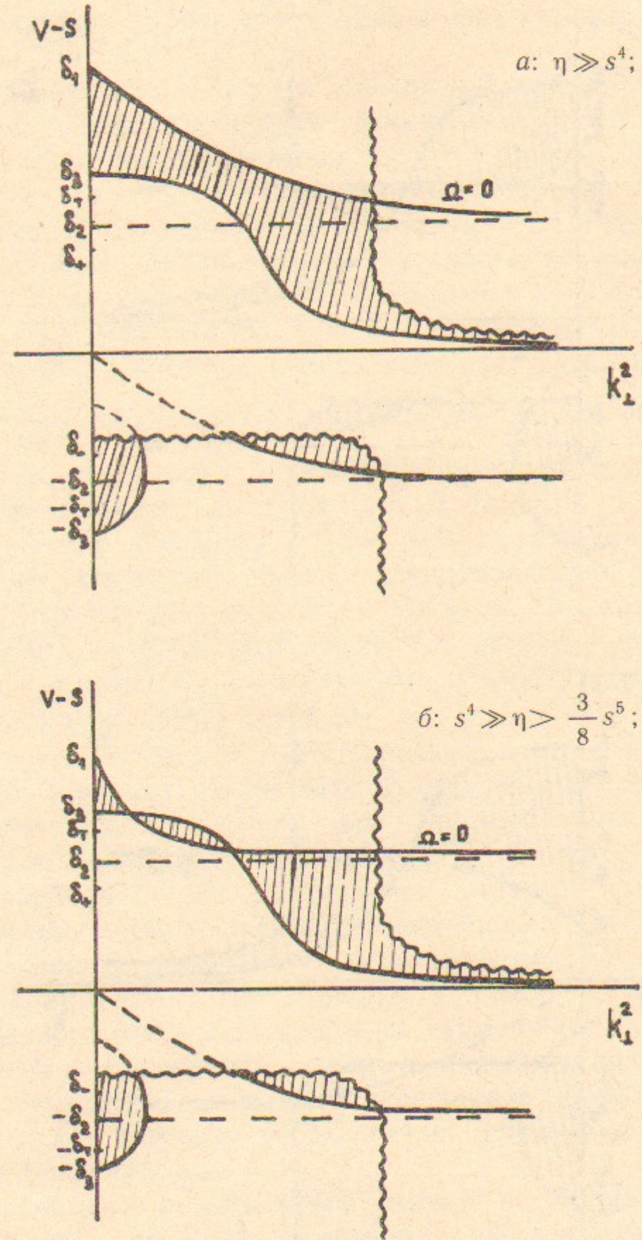
Рис. 2. Характер линейной устойчивости в пространстве (v-s) - k_{\perp}^2 . Заштрихованная область неустойчива. Волнистые линии ограничивают области, где решение (7) не определено. \delta_1 = 4\eta/s^3 , \delta_2 = \sqrt{3\eta/4} , \delta_3 = \sqrt{3}/2 \cdot \sqrt{\eta/s} , \delta_{\pm} = \pm\sqrt{\eta/2} .
